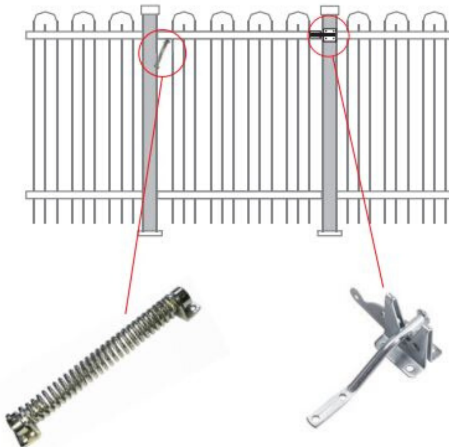
Ressort et loquet en acier inoxydable pour porte simple à fermeture automatique
